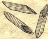
Pennes
